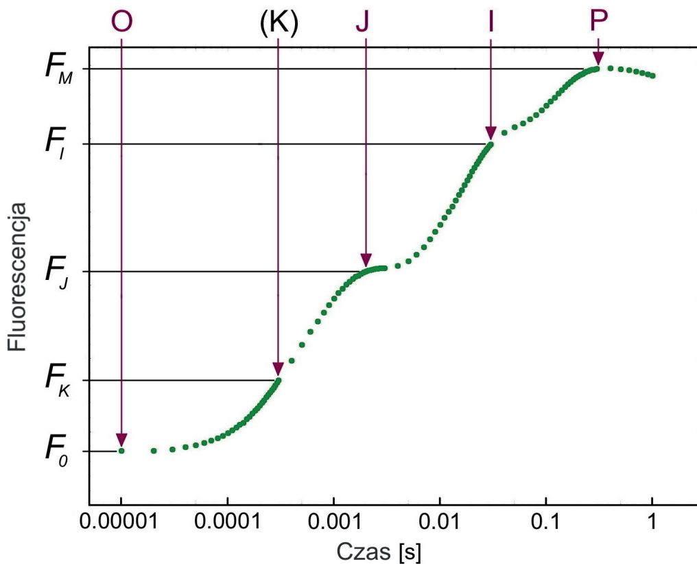
Ryc. 7. Krzywa indukcji fluorescencji otrzymana z fluorymetru typu PEA, po adaptacji próbki w ciemności, a następnie naświetleniu silnym światłem aktywnym. F_0 – fluorescencja minimalna w stanie zaadaptowania do ciemności, F_m – fluorescencja maksymalna w stanie zaadaptowania do ciemności, O(K)JIP – kolejne stopnie wyznaczone umownie na krzywej fluorescencji: O= F_0 , K przy 300 \mu s, J przy 2 ms, I przy 30 ms, P= F_m . Wielkość fluorescencji podawana jest w jednostkach względnych, przyjętych przez producenta urządzenia. (TS)
