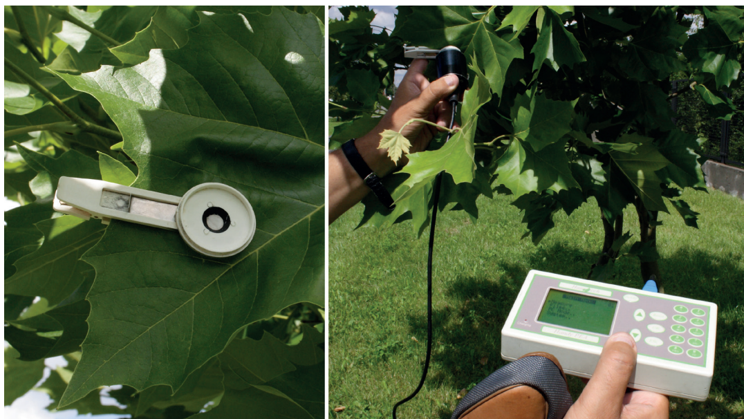
Ryc. 9 (po lewej): Specjalny klips z zasuwką umieszczony na liściu w celu adaptacji do ciemności, producent: Hansatech Instruments Ltd., Kings Lynn, UK. (TS)
